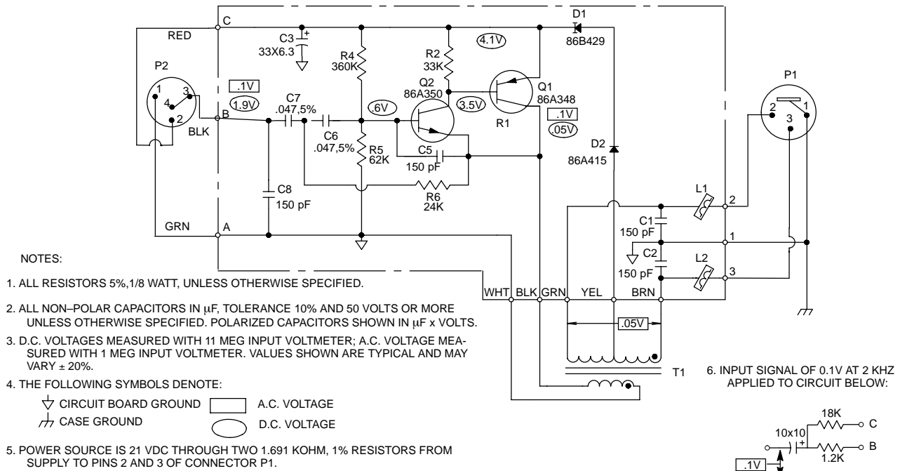
SCHÉMA DE PRINCIPE DU PRÉAMPLIFICATEUR SM93 • STROMLAUFPLAN FÜR VORVERSTÄRKER SM93 • DIAGRAMA ESQUEMATICO DEL PREAMPLIFICADOR SM93 • SCHEMA CIRCUITALE DEI MODELLI DEL PREAMPLIFICATORE SM93 FIGURE 5
